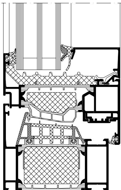
Wärmedämmung auf Passivhausniveau, Maßstab 1:2 Thermal insulation to passive house level, Scale 1:2
