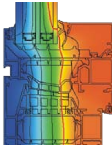
Schüco Fenster AWS 90.SI+, Maßstab 1:2 Schüco Window AWS 90.SI+, Scale 1:2
